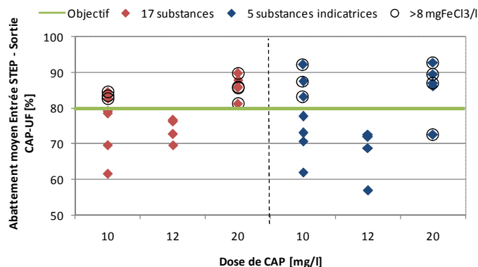
Figure 60 : Influence du dosage de CAP sur l'abattement moyen de 17 substances (cf. annexe 7) (à gauche), ou des 5 substances indicatrices (à droite), entre l'entrée de la STEP et la sortie du traitement CAP-UF. Résultats basés sur 16 analyses (représentées chacune par un point).
