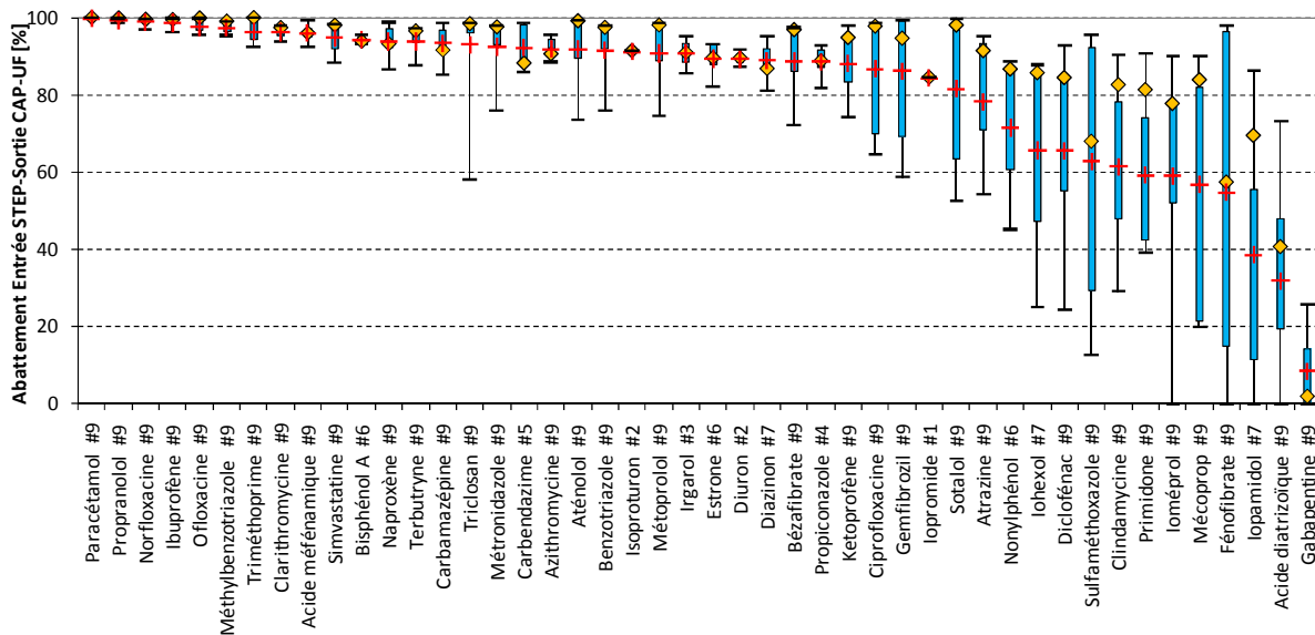
Figure 28 : Abatement de 46 micropolluants détectés entre l'entrée de la STEP et la sortie de l'installation CAP-UF (y compris l'effet du traitement biologique) lors de 3 GC (9 analyses, dosage de CAP entre 10 et 20 mg/l). Le numéro (#) indique le nombre d'analyses pour la substance. Représentation avec les quartiles 25-75% (rectangle bleu), les valeurs minimum/maximum et la moyenne (+). Le losange orange (◊) représente la moyenne de la GC de mai, lors de laquelle le traitement CAP-UF était optimisé (20 mgCAP/l, 88% d'élimination sur les 46 substances). (L'abatement moyen des 46 micropolluants sur les 3 GC est de 82%)
