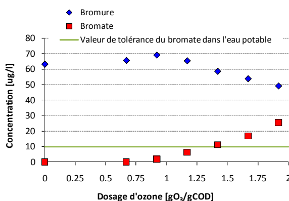
Figure 33 : Influence du dosage d'ozone sur la formation de bromate (ozonation de l'effluent du LF en nitrification totale, 5 mgCOD/l, 0.6 mgN-NO 2 /l. Expérience réalisée à l'Eawag, département W+T). A faible dose (<1 gO 3 /gCOD), l'oxydation du bromure en bromate est négligeable à cause de la consommation rapide de l'ozone par le nitrite et le COD réactif. Au-dessus de 0.9 gO 3 /gCOD, on observe une relation linéaire entre le dosage et la formation de bromate (également observée dans l'étude de Wert et al. (2007)).
