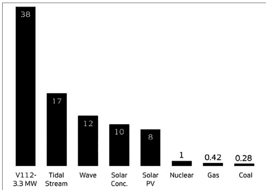
[Fig. 16 - Comparatif du taux de retour énergétique de différentes sources d'énergie.]
