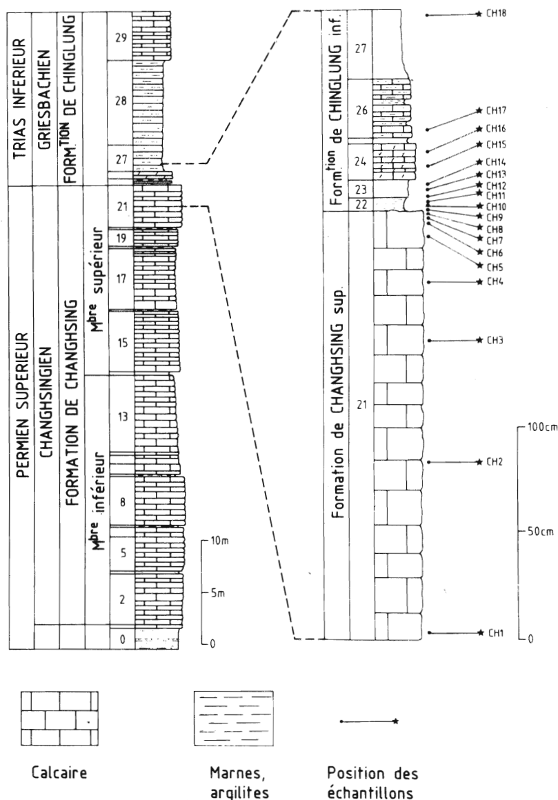
Colonne stratigraphique de la coupe de Meishan, Changhsing.
