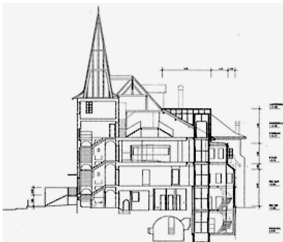
Figure 8 : Une coupe transversale montre l'organisation et accès aux étages ici dénommés -rez inf., rez sup., étage et combles (ACV). Un escalier en colimaçon permet, depuis l'entrée à la rue Saint-Etienne no 7, l'accès aux étages inférieurs, avec l'auditoire, les collections et expositions.
