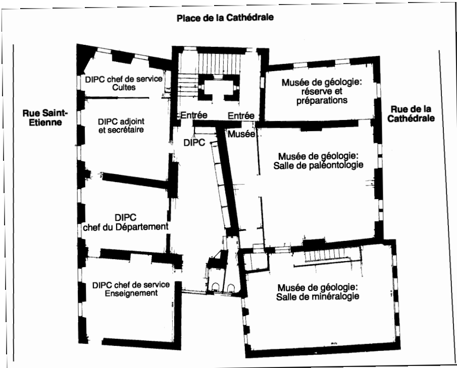
Figure 6 : plan du deuxième étage (doc. ACV complété) avec l'agencement.
