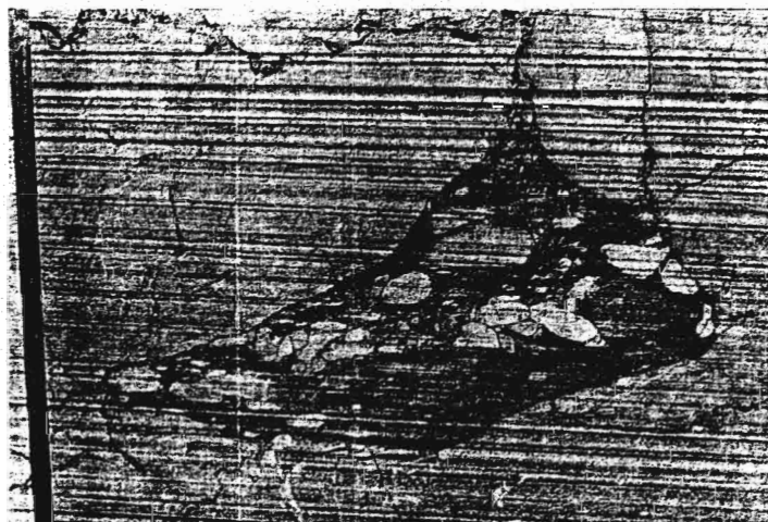
Fig. 4. Conduit karstique avec remplissage granoclassé complexe (série renversée).
